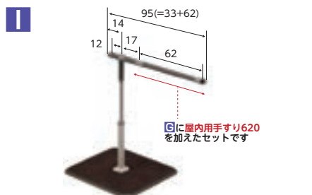
屋内用回転手すり330+620
