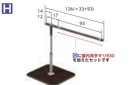
屋内用回転手すり330+930
