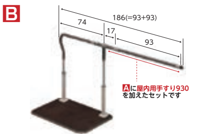
屋内用930タイプ+930
